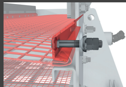
SCHRAUBBEFESTIGUNG
